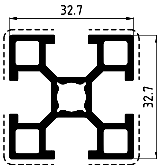
PROFILO BINARIO DFV0913 0,794 Kg/ml
