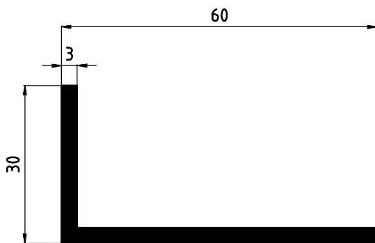
ELLE BST0918_SM 0,705 Kg/ml
