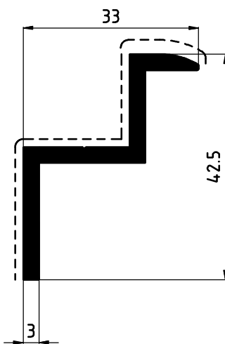
STAFFA LATERALE DFV0914 0,575 Kg/ml
