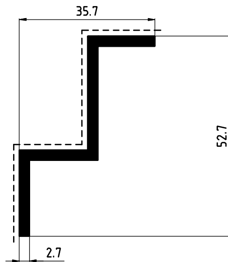
STAFFA LATERALE DFV1222 0,624 Kg/ml
