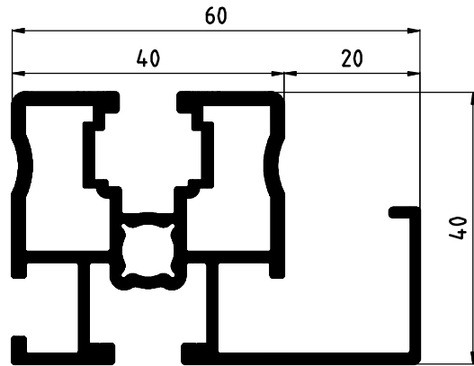
PROF. STRUTTURALE DFV0912_SM 1,310 Kg/ml
