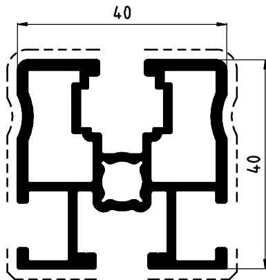
PROF. STRUTTURALE DFV0911 1,148 Kg/ml
