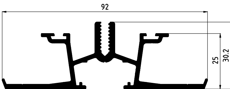
SUPPORTO PANNELLI DFV0920 1,138 Kg/ml
