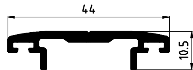
PRESSORE DFV0919 0,377 Kg/ml
