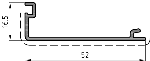
BBC1483 24862 0.307 Kg/m CARTELLA INCONTRO CENTRALE
