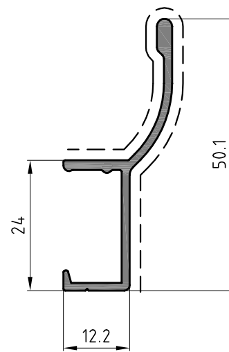
BBC1485 24864 0.335 Kg/m CARTELLA RACCOGLICONDENSA
